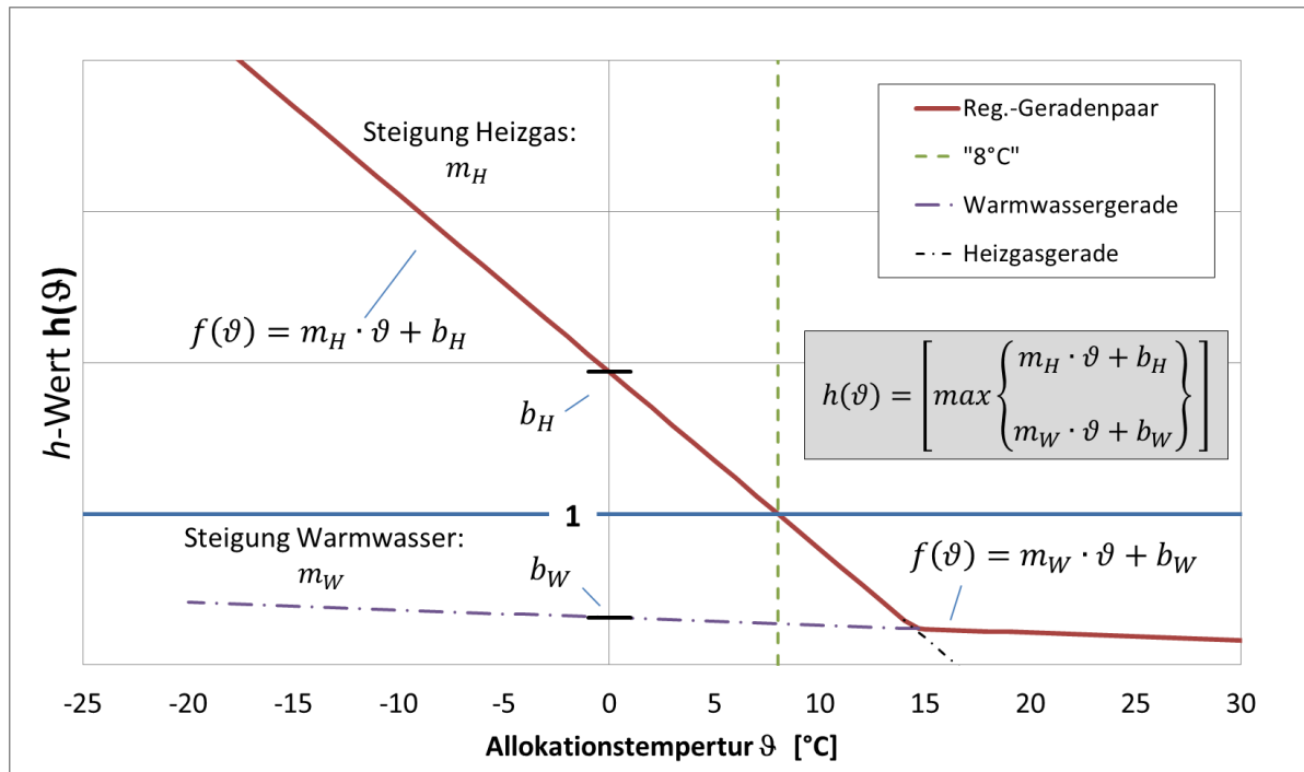
Abbildung 31 Wirkungsweise Regressionsgeradenpaar
