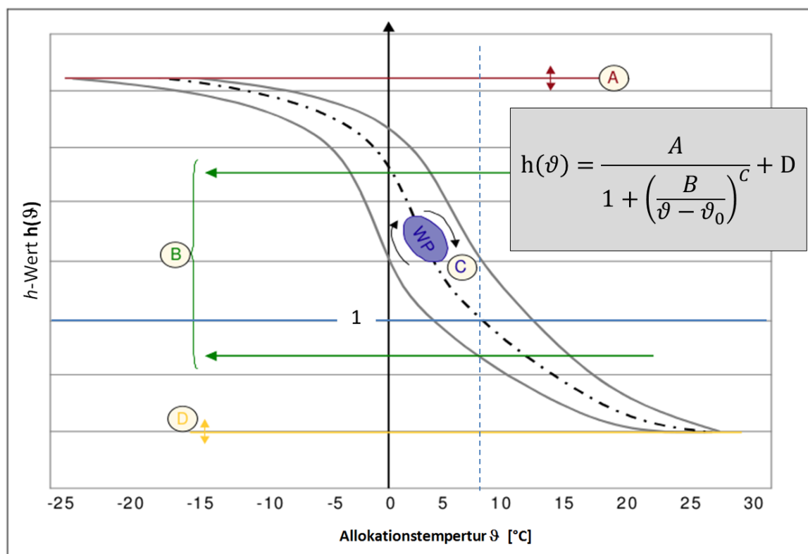
Abbildung 30 Wirkungsweise Sigmoid-Funktion
