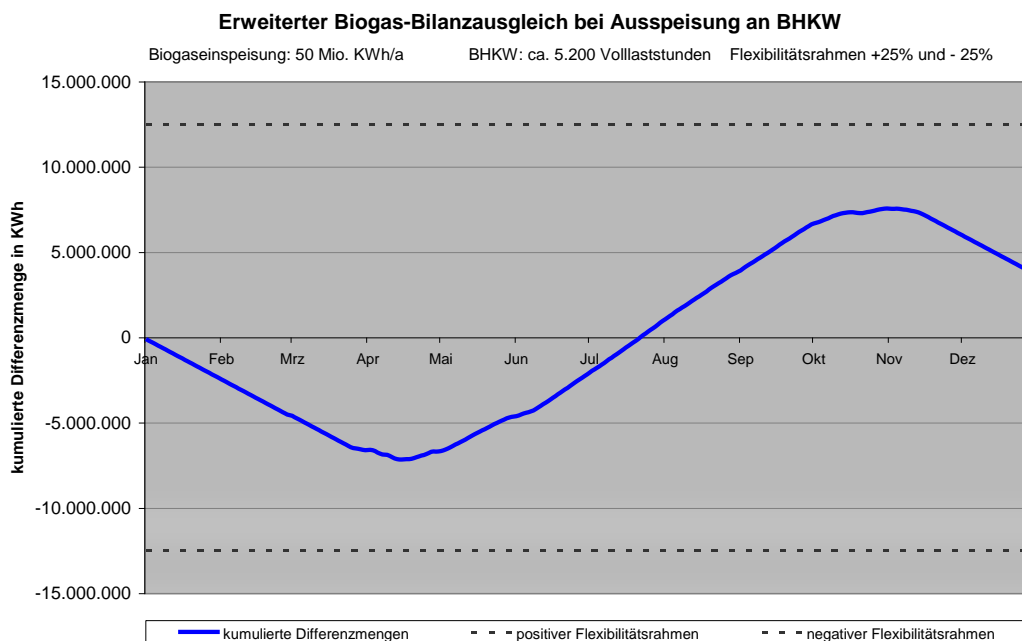
Abbildung 2 Erweiterter Biogas-Bilanzausgleich bei Ausspeisung an BHKW
