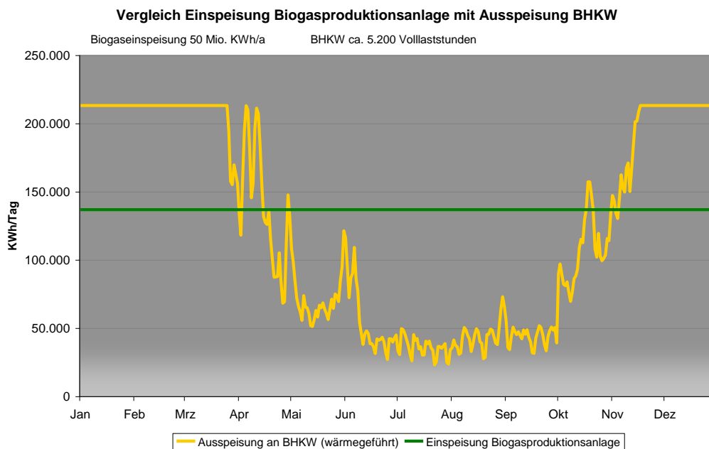
Abbildung 1 Beispiel für die Einspeisung aus einer Biogasproduktionsanlage und der Ausspeisung an ein BHKW 1
