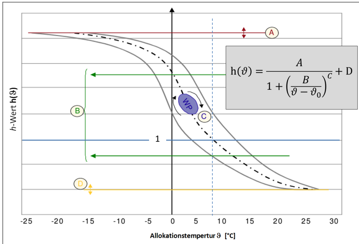
Abbildung 32 Wirkungsweise der Sigmoid-Funktion
