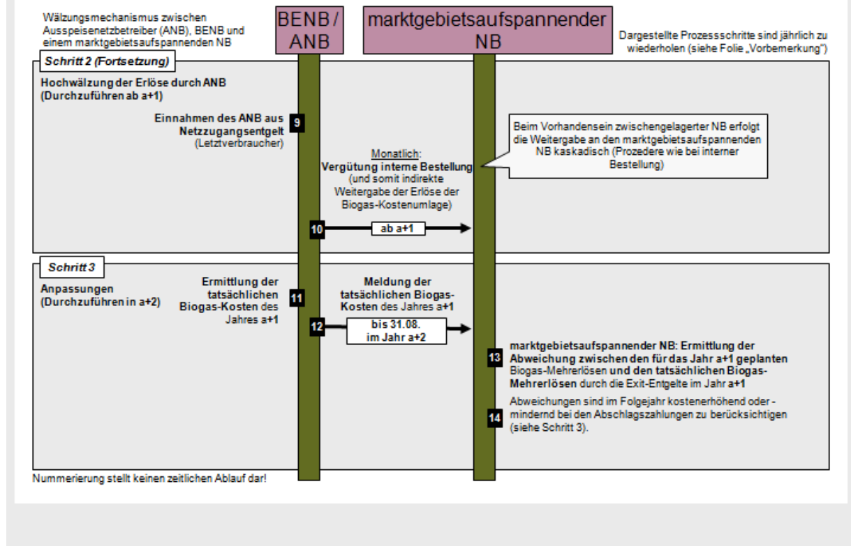
Abbildung 6 Wälzungsmechanismus Biogas - interne Bestellung (Bild 2)
